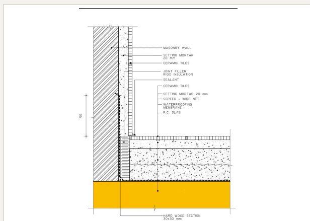
تفاصيل تنفيذية
